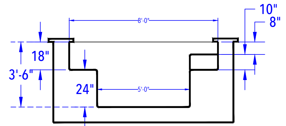
SPA ELEVATION N.T.S
